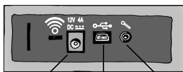
DC Socket MINI USB Socket External Microphone
